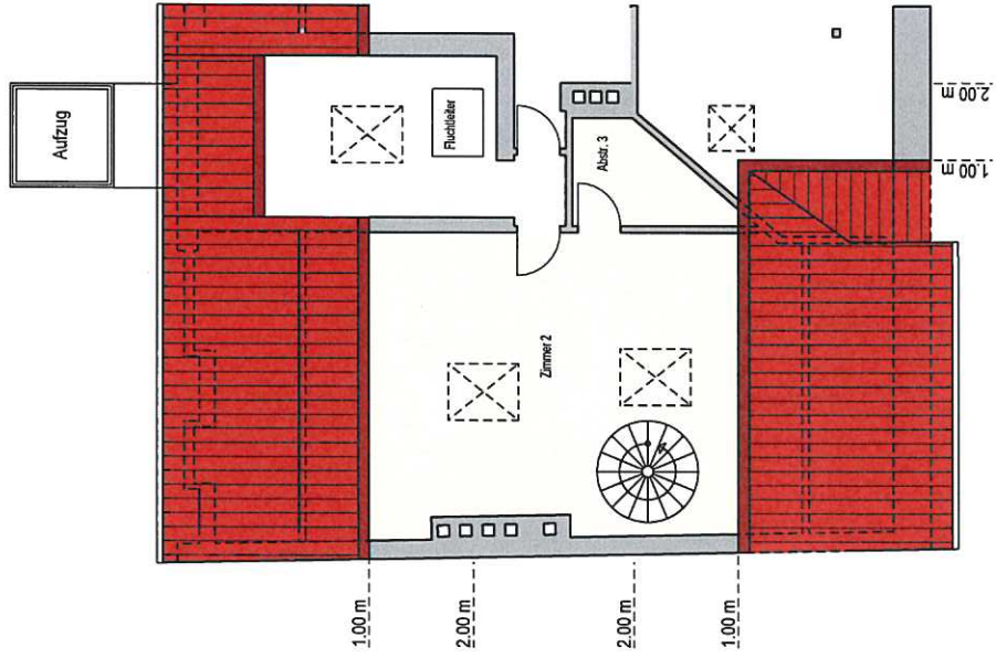
Dachgeschoss 2
