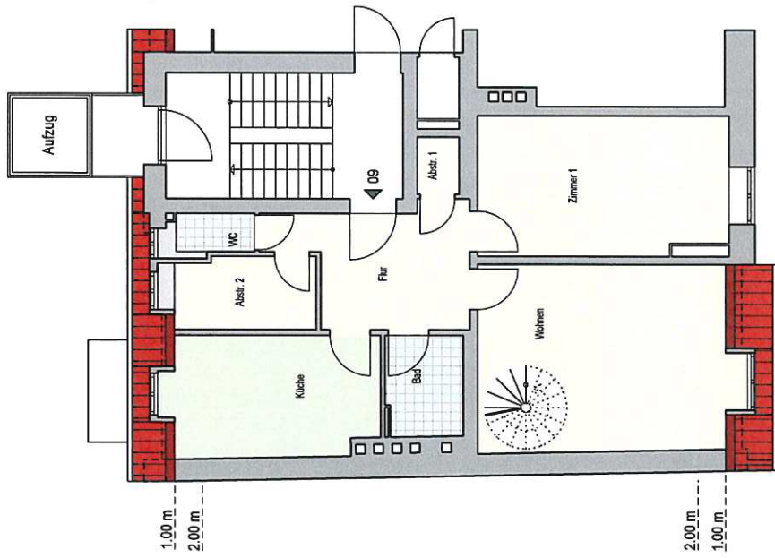
Dachgeschoss 1
